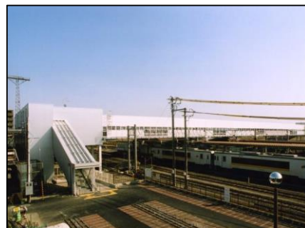
【JR小牛田駅自由通路】 □場所: 宮城県遠田郡美里町 □竣工年: 2006/3
